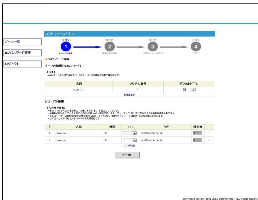
4-2 正引き/逆引きの各ゾーンの編集トップ画面
