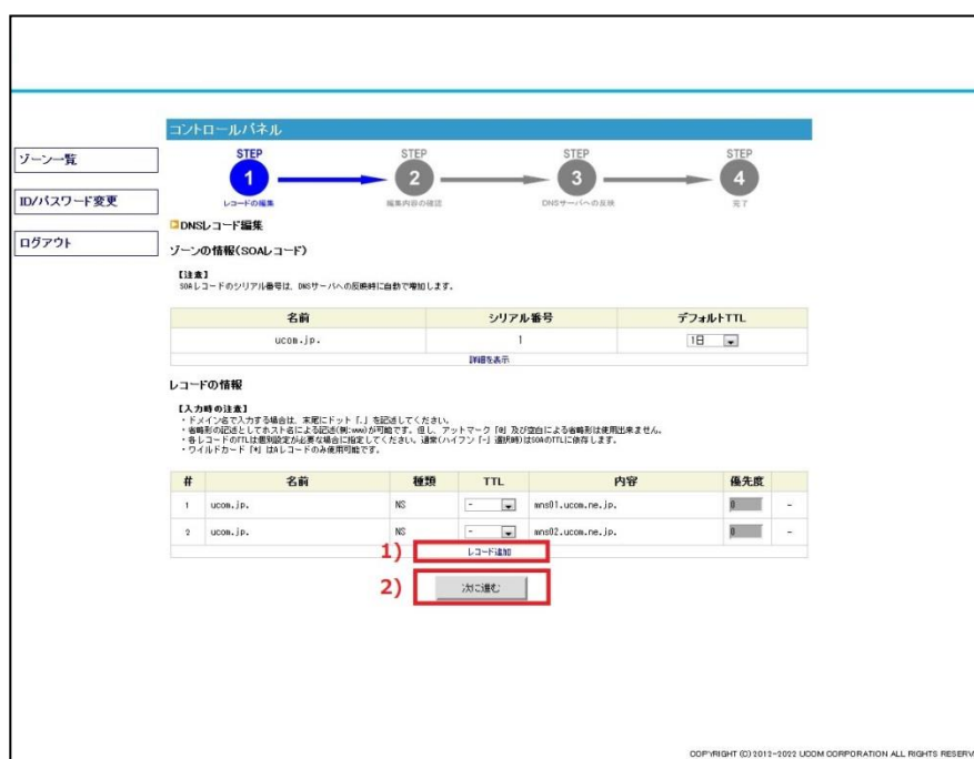
図 4-3 「レコード追加」リンク箇所
